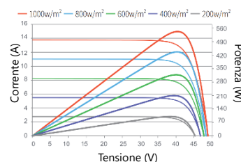
Curva corrente-tensione e potenza-tensione (540W)
