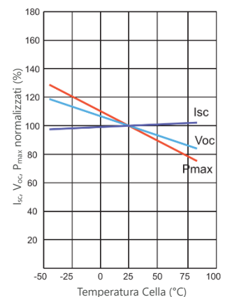
Dipendenza dalla temperatura di I sc , V oc , P max
